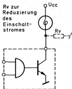
Lampentreiber
