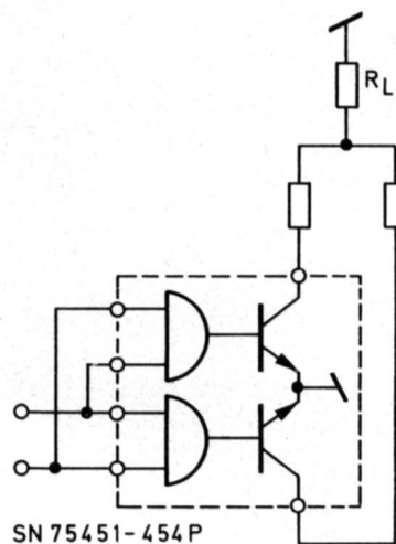
600 mA-Treiber
