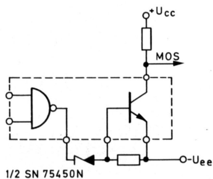
300 mA-Leistungsschalter mit variablem Bezugspotential
